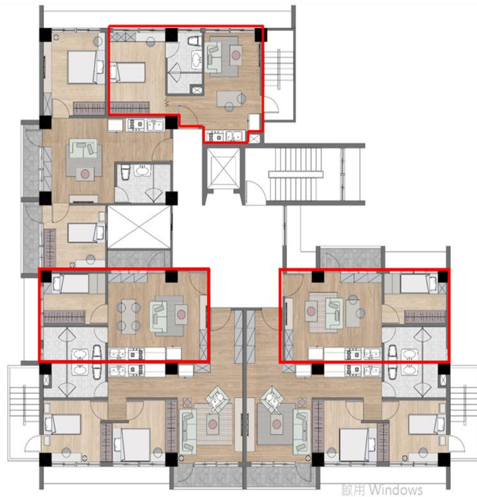
9樓整修平面規劃及家配圖(3間套房, 3間雙房間)
