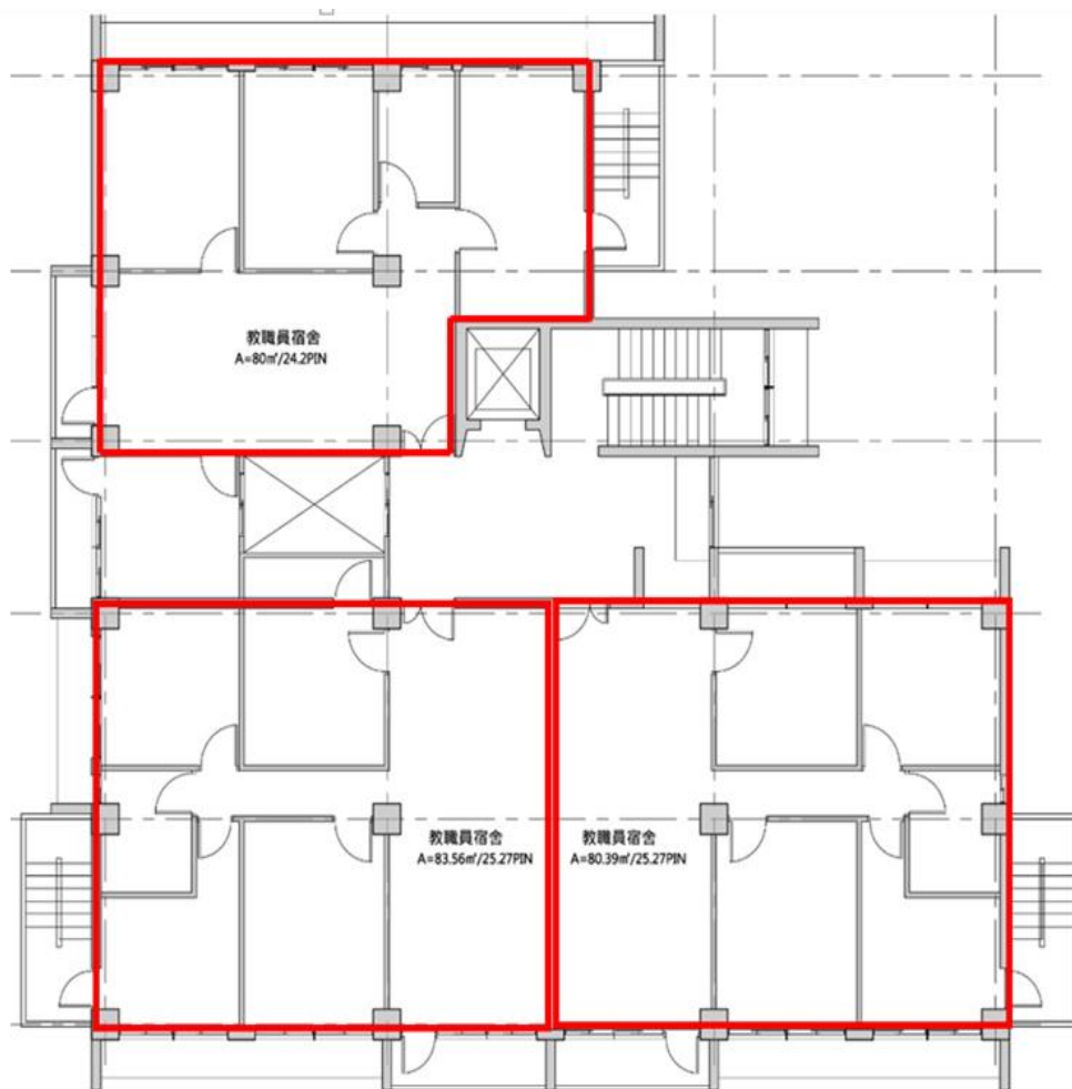
9樓現況平面圖(3間3房間)
